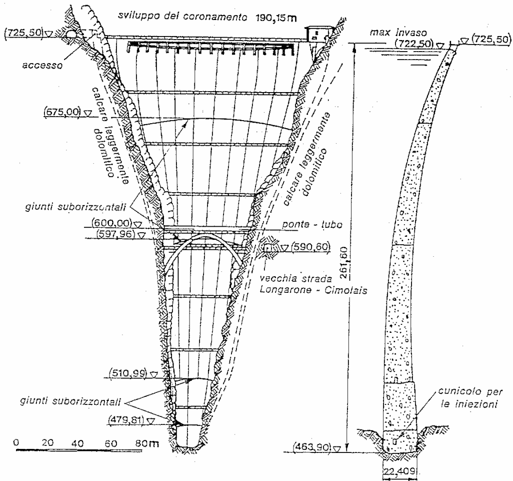
Fig. 3-3. Diga ad arco del Vajont [73].
