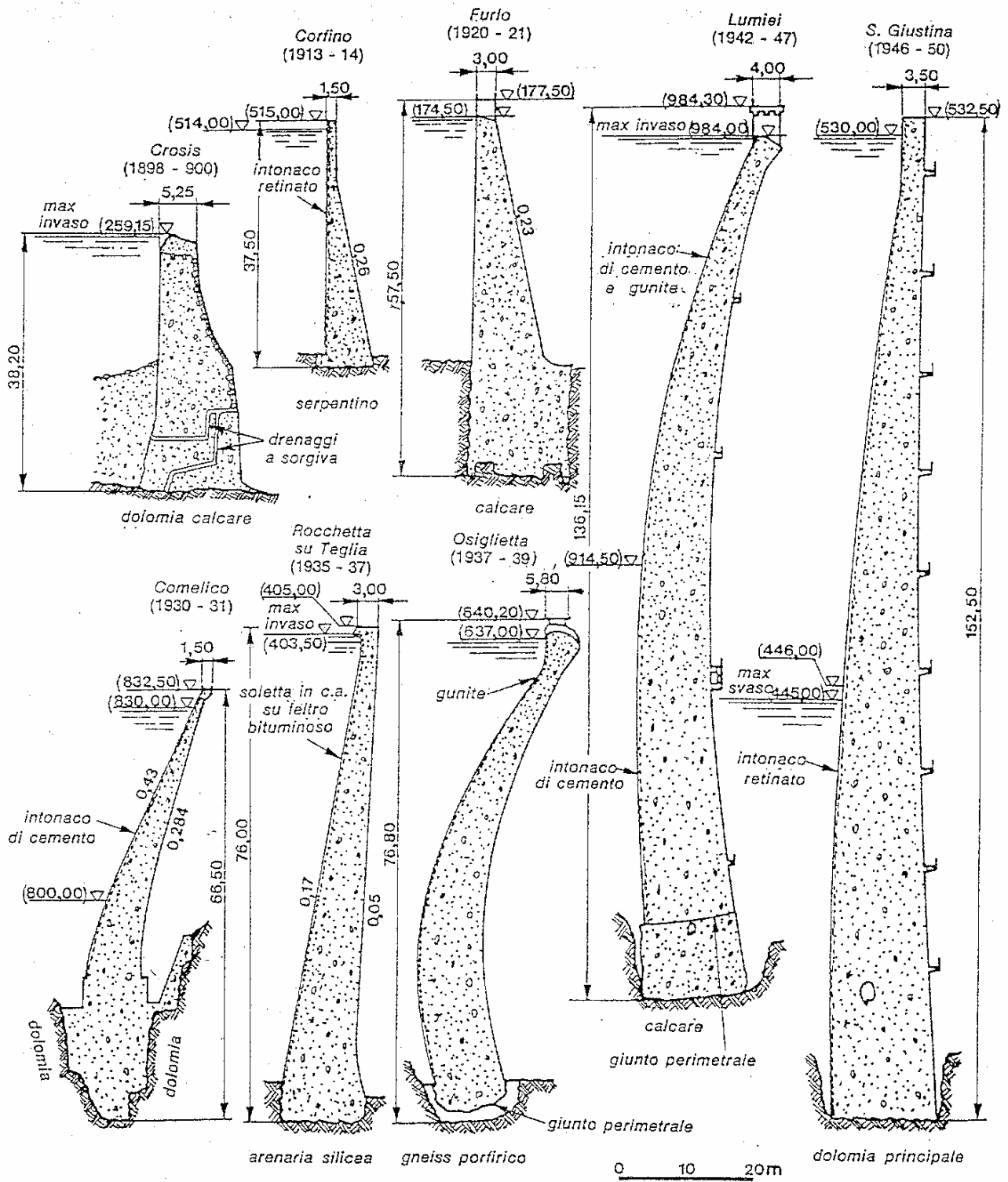
Fig. 3-2. Sezioni maestre di dighe spingenti italiane [73].
