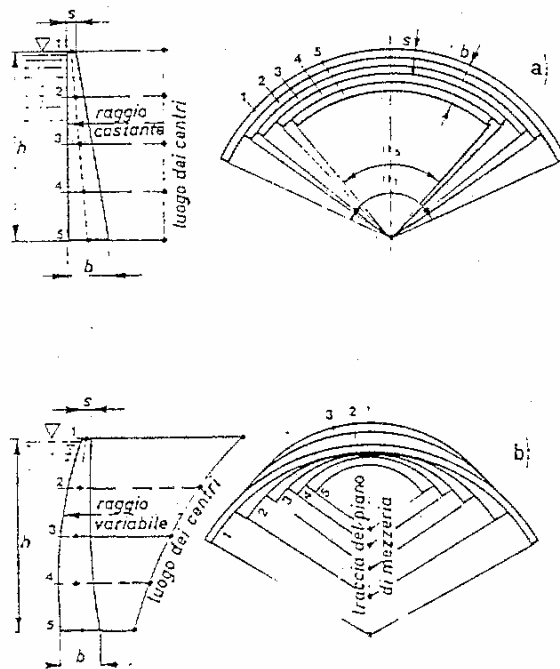
Fig. 3-1. Configurazioni geometriche limiti delle dighe spingenti: a) diga a raggio costante; b) diga ad apertura costante [91].
